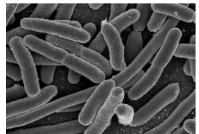
大肠杆菌
